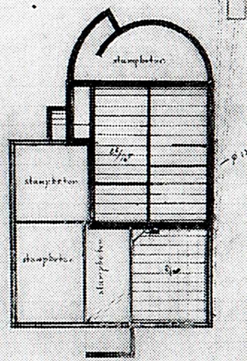
vloerligging
