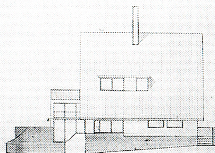
NO gevel
