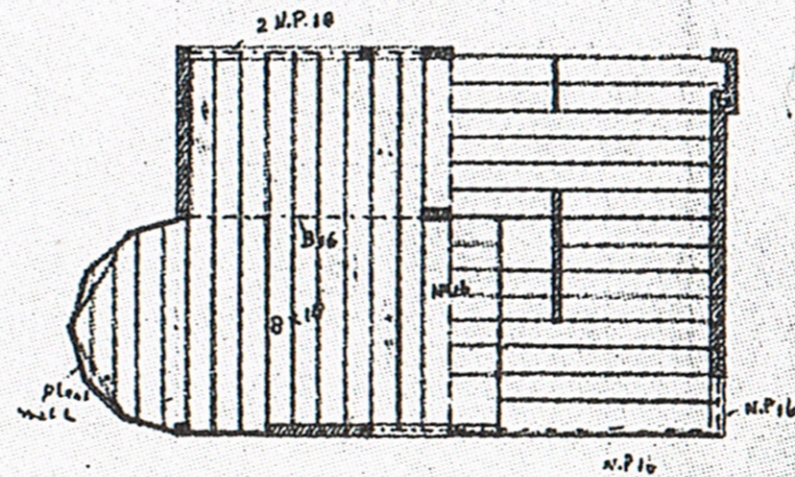
2e balklaag
