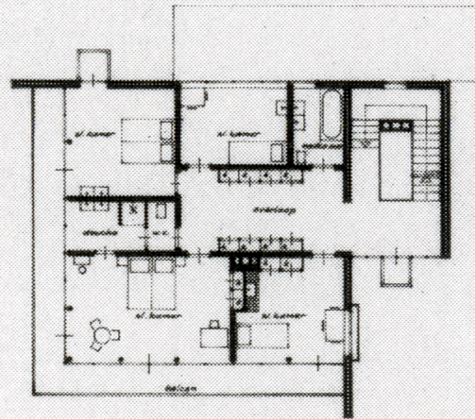
VERDISPING
