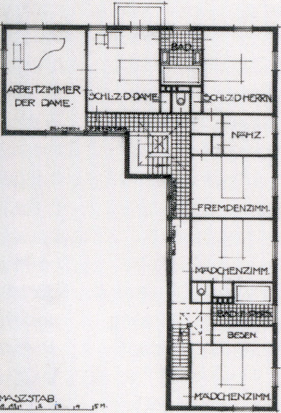
OBERGESCHOSS.
