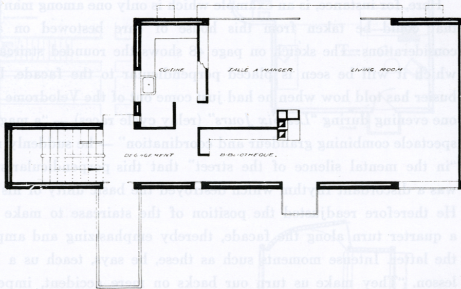
Rez-de-chaussée haut
