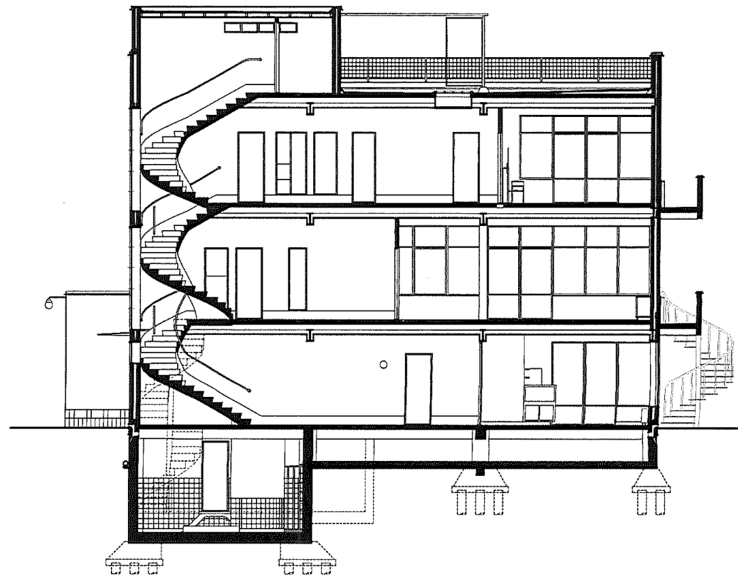
Longitudinal section
